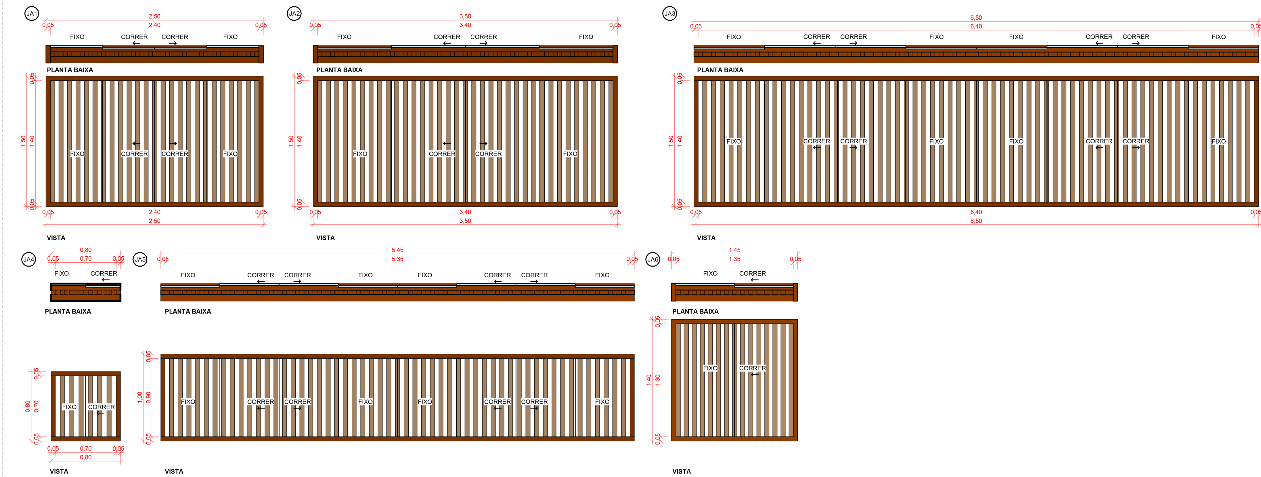
DET. 30 - JANELAS - PADRÃO INDÍGENA
