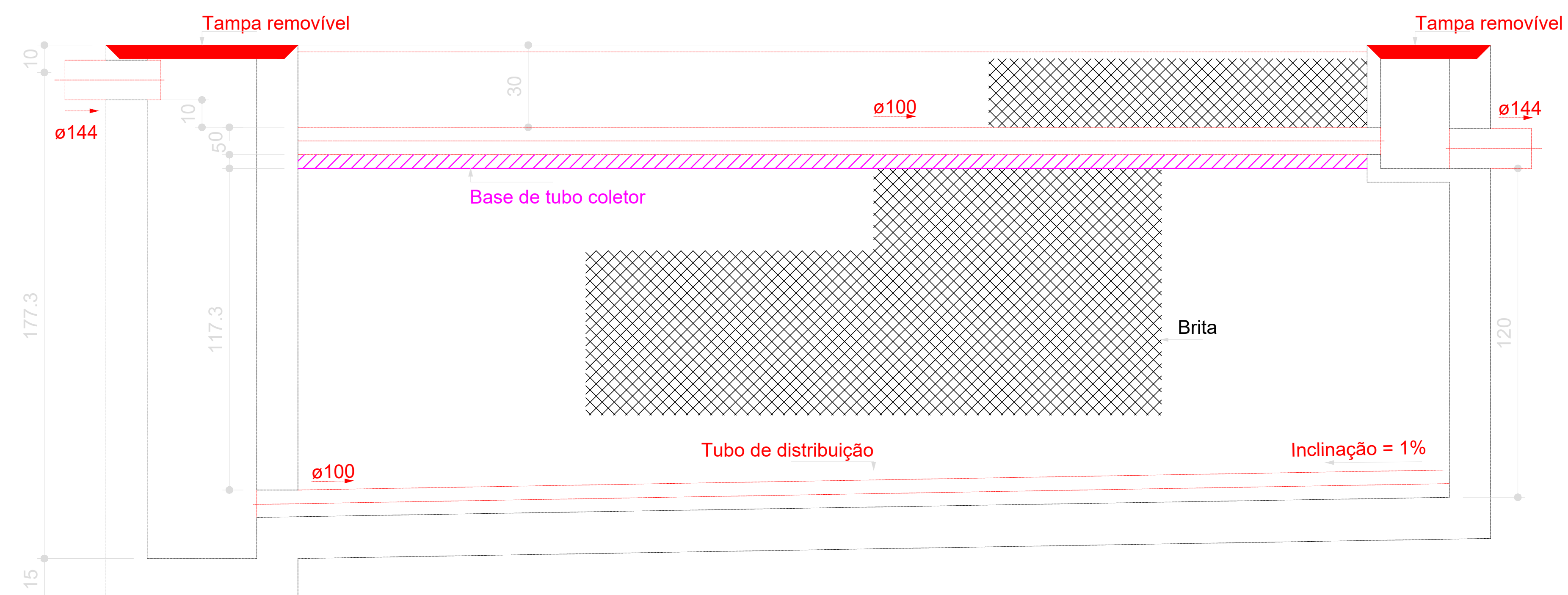
Filtro anaeróbio - TÉRREO Corte 1 - ESC. 1:25
