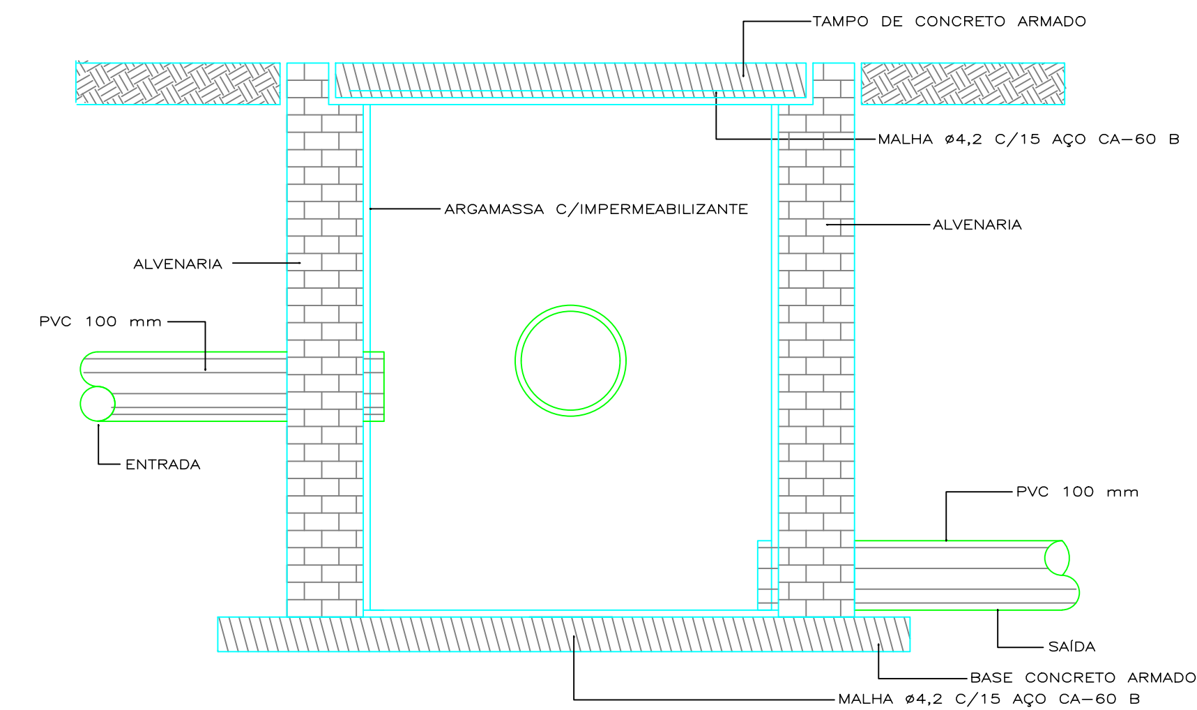
CORTE A.A-s/esc
