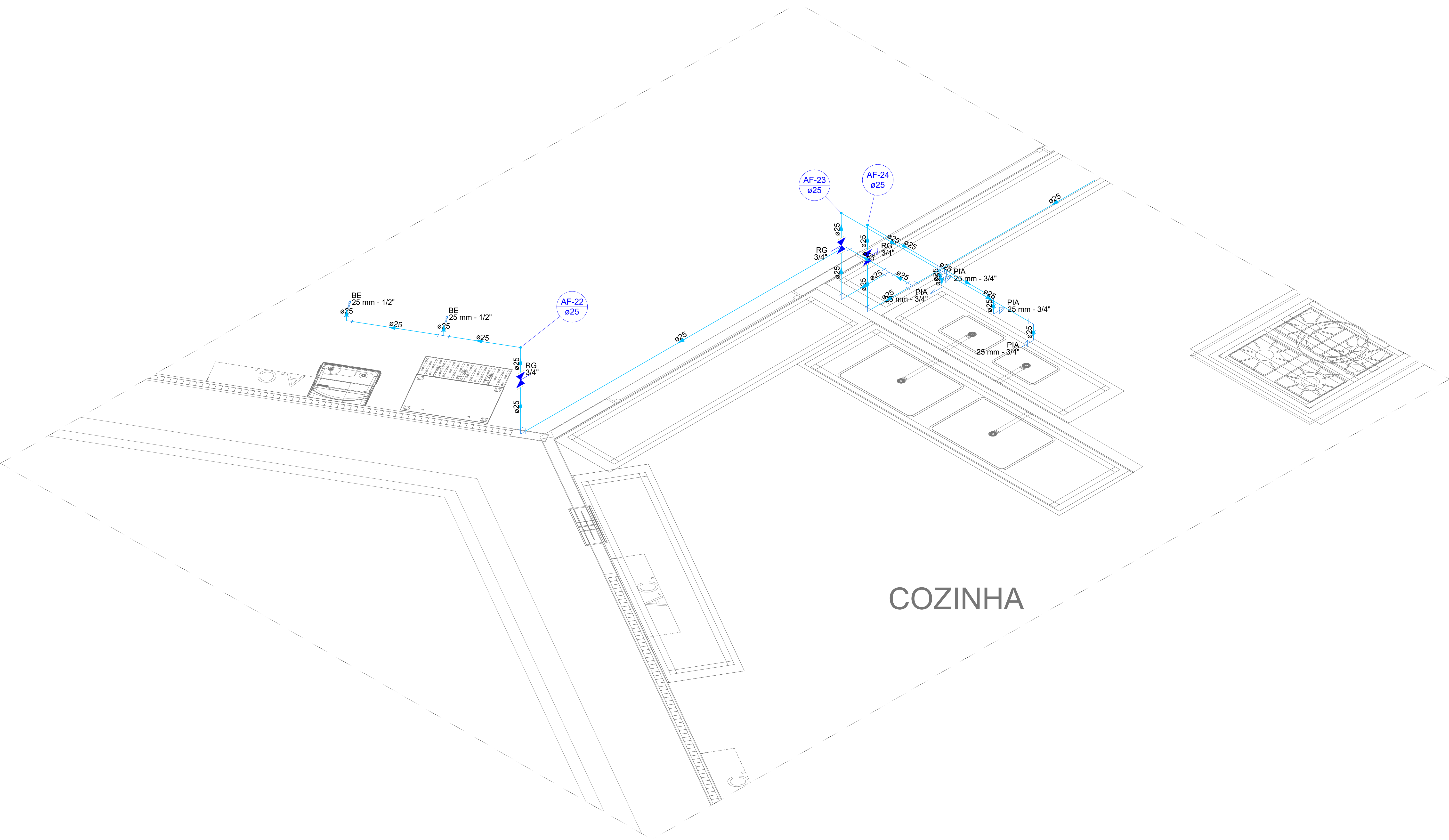
4 Detalhe Isométrico HID-5 ESCALA: 1/25
