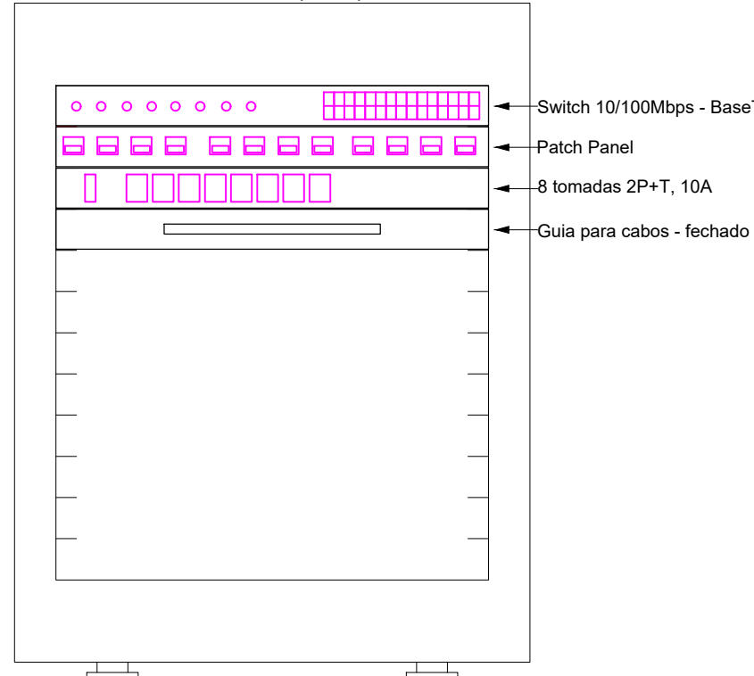
Plano de face do rack (BD1) - Pavimento
