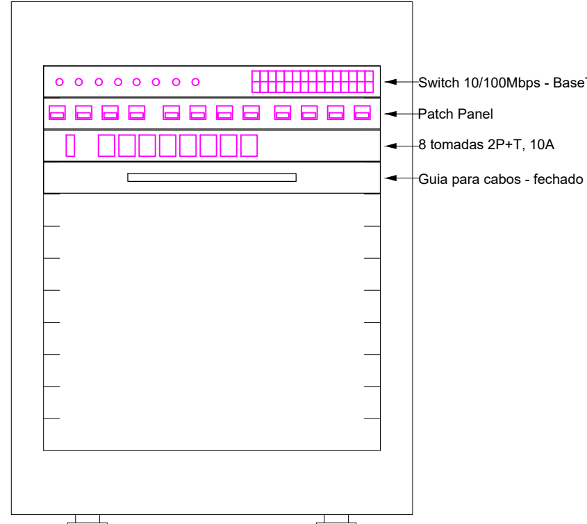
Plano de face do rack (FD1) - Pavimento
