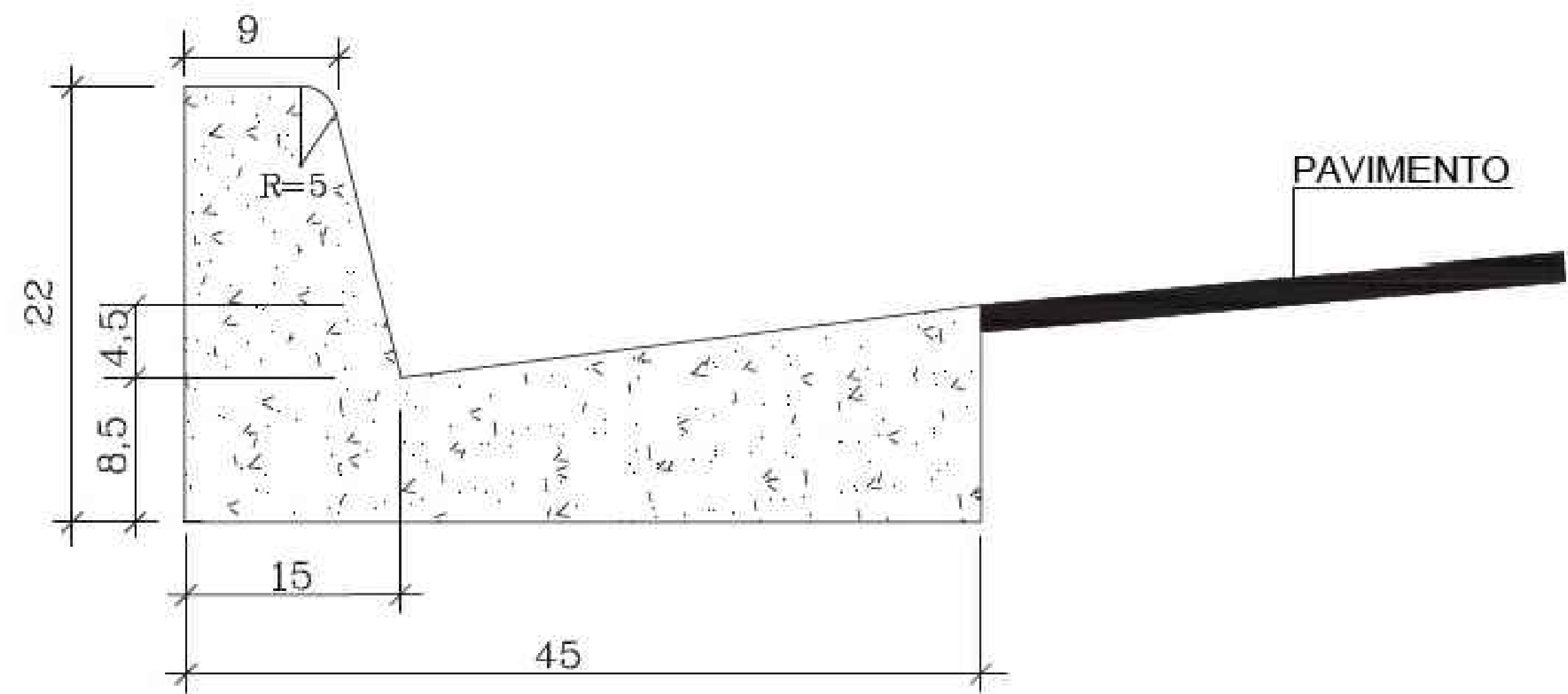
DETALHE DO MEIO FIO E SARJETA
