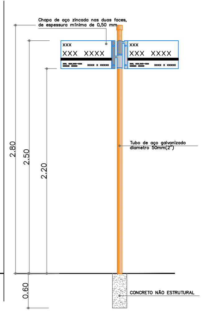
DETALHE FRONTAL
